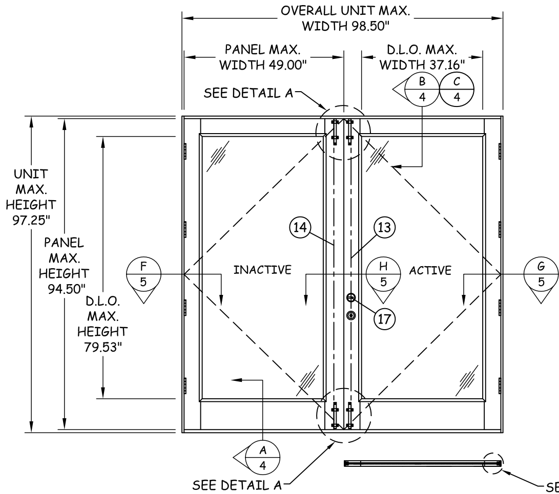
ELEVATION
